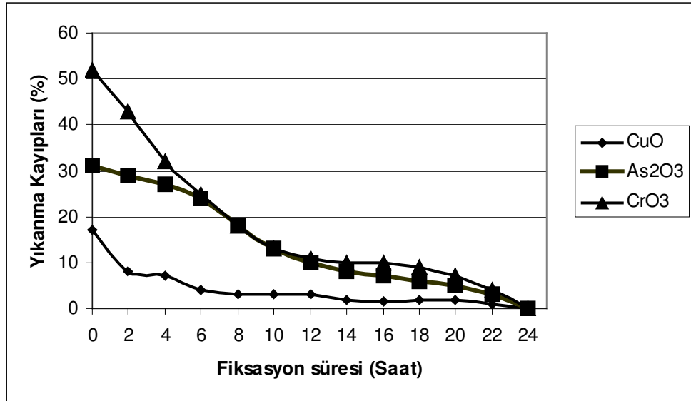
Şekil 1. CCA ile empenye edilmiş ve 45°C'de fiksasyon işlemi tamamlamış odun örneklerinde meydana gelen yıkanma kayıpları (6).
